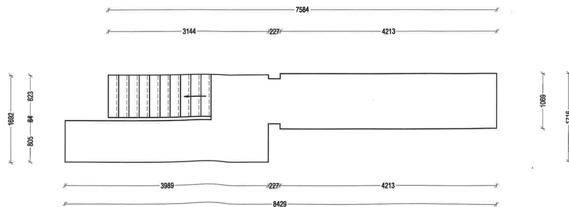
GRONDPLAN VERDIEPING -1
