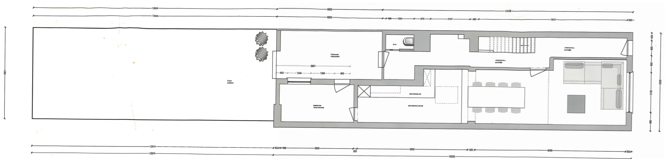
GRONDPLAN GELIJKVLOERS
